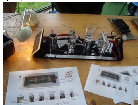
Figure 4 : Maquette d'une pile à combustible
